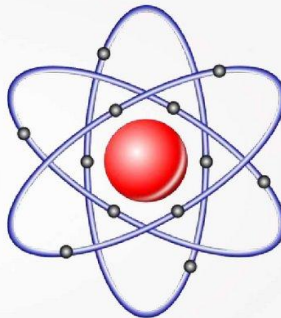
Планетарная модель атома Резерфорда
